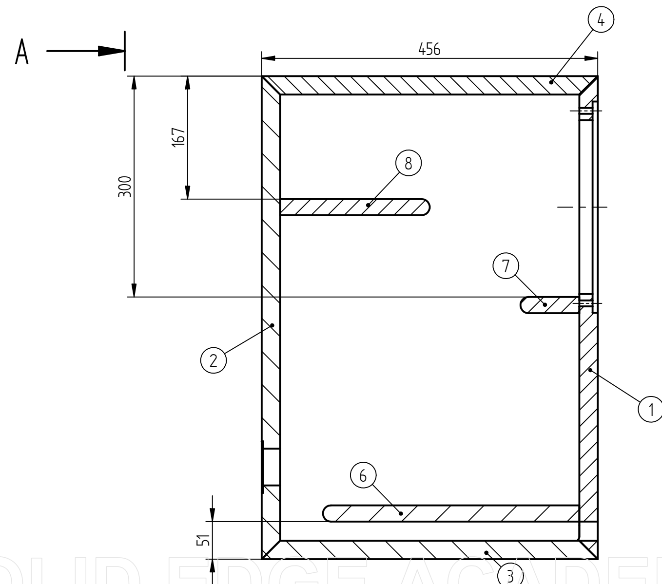
Schnitt A-A
